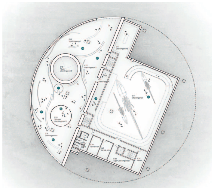
1. Untergeschoss M. 1.000
