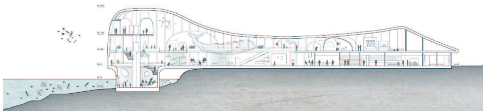
Schnitt A-A M. 1.000
