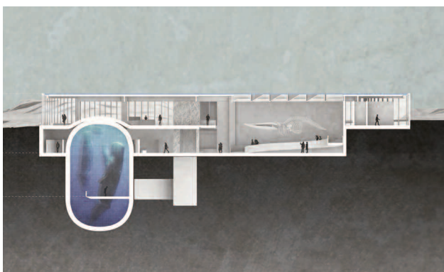
Schnitt M. 1.000
