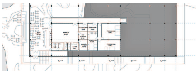
Untergeschoss M. 1.000
