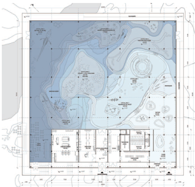
Erdgeschoss M. 1.000
