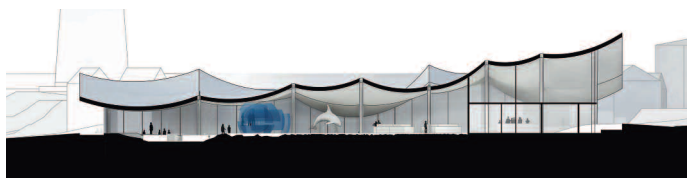
Schnitt A-A M. 1.000
