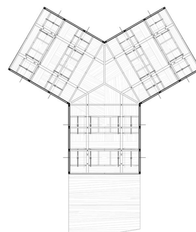
Grundriss
