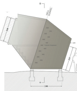
SEITENANSICHT M. 1:200
