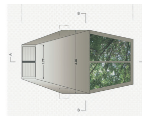
DACHAUFSICHT M. 1:200
