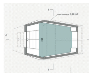
GRUNDRISS UNTEN M. 1:200
